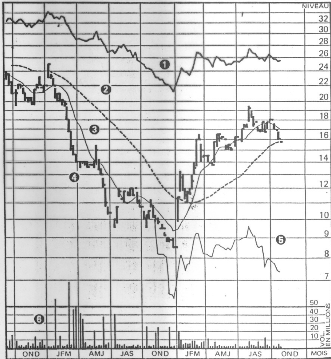
Graphique type. En 1 on trouve la courbe de variation relative, en 2 la courbe de la moyenne mobile à 200 jours, en 3 la courbe de la moyenne mobile à 50 jours, en 4 l'évolution des cours de la valeur, en 5 la courbe de on-balance-volume et en 6 les volumes de transaction.
